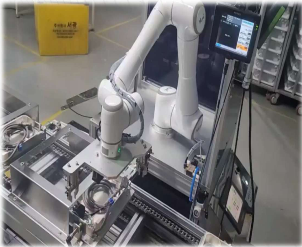
취출 및 비전 검사 (전자품)
